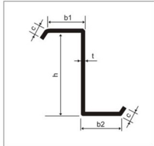
Z型钢檩条规格尺寸表 Z purlin dimensions table
